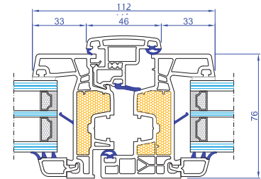
Nodo centrale asimmetrico
