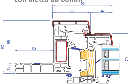
Telaio da ristrutturazione con aletta da 60mm
