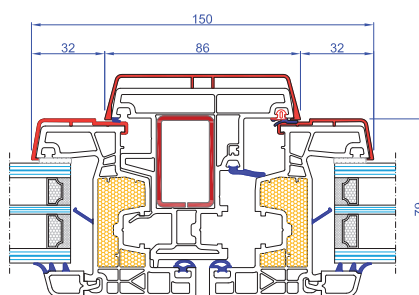
Nodo centrale simmetrico
