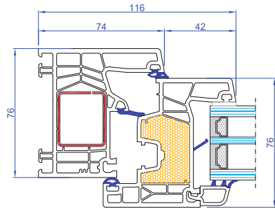
Telaio a "L"
