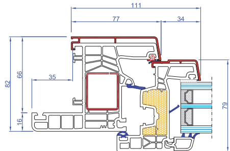
Telaio con aletta da 35mm
