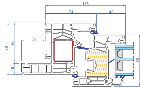
Telaio con aletta da 35mm
