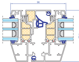
Nodo centrale Asimmetrico
