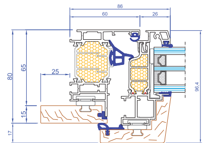
Telaio con aletta da 25mm
