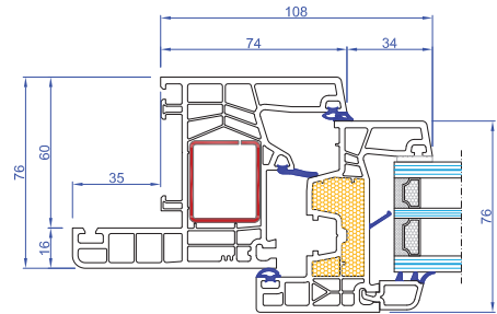
Telaio con aletta da 35mm
