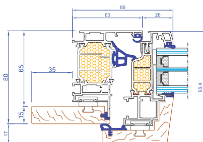
Telaio con aletta da 35mm
