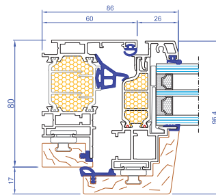
Telaio a "L"
