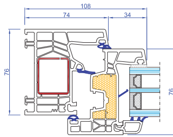
Telaio a "L"
