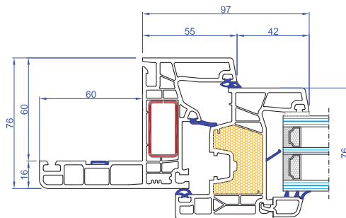
Telaio da ristrutturazione con aletta da 60mm
