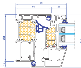
Telaio a "L"
