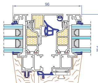
Nodo centrale Asimmetrico
