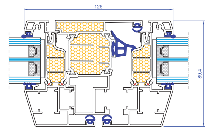
Nodo centrale Simmetrico
