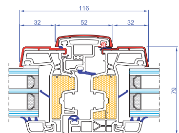
Nodo centrale asimmetrico
