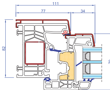
Telaio a "L"
