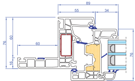
Telaio da ristrutturazione con aletta da 60mm
