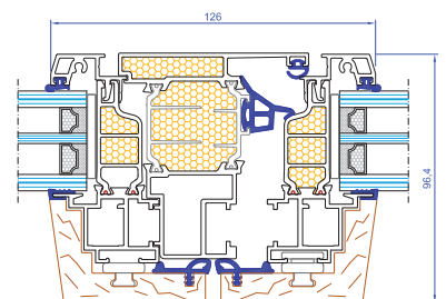
Nodo centrale Simmetrico
